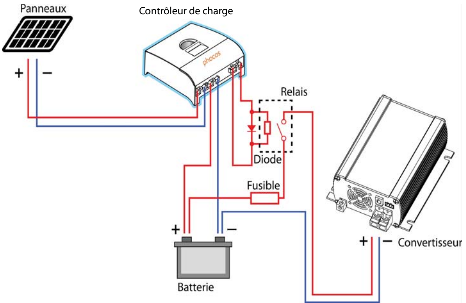
Diagramme électrique pour un système photovoltaïque utilisant un contrôleur de charge
