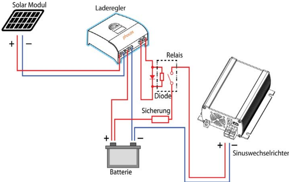
Schaltplan für eine PV-Anlage mit Laderegler
